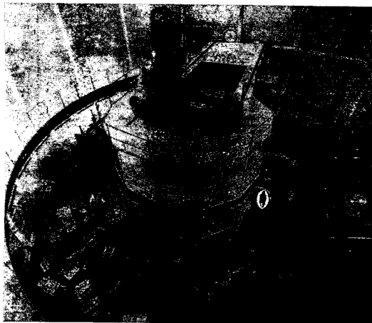
Forskningsreaktoren JEEP II ved IFA's anlegg på Kjeller.
